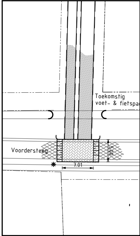
Plateau toekomstg voet-en fietspad
