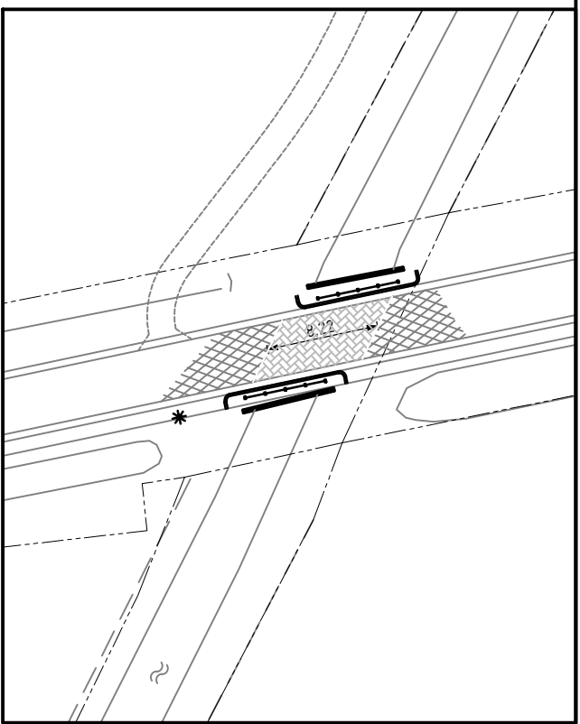
Nieuwe komgrens +toekomstg fietspad Fliet
