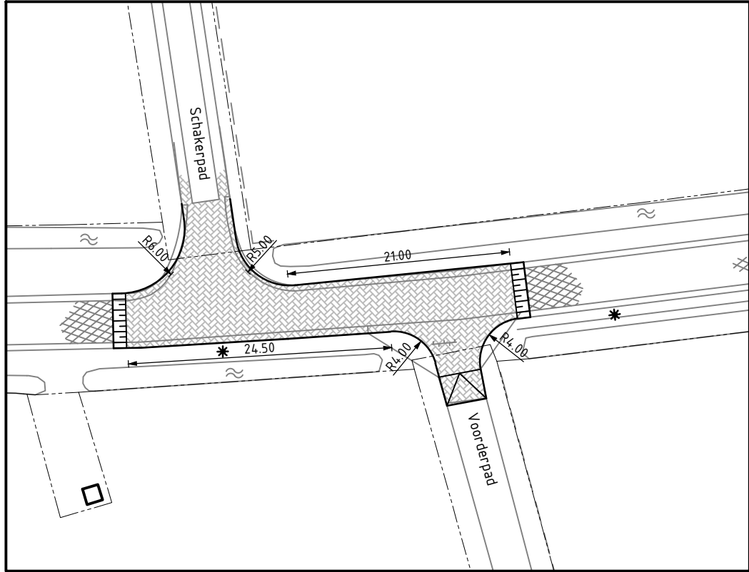
Verlengd plateau Voorderpad/Schakerpad/Voordersteeg
